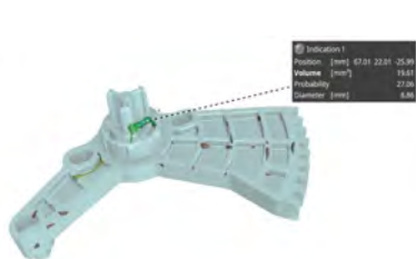
Analýza pórovitosti/vnitřních defektů
