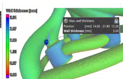
Analýza tloušťky stěn
