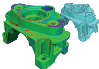
Srovnání vyrobeného dílu s jeho 3D modelem
