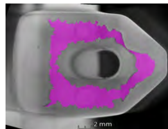
Kontrola svarů/montáže sestav
